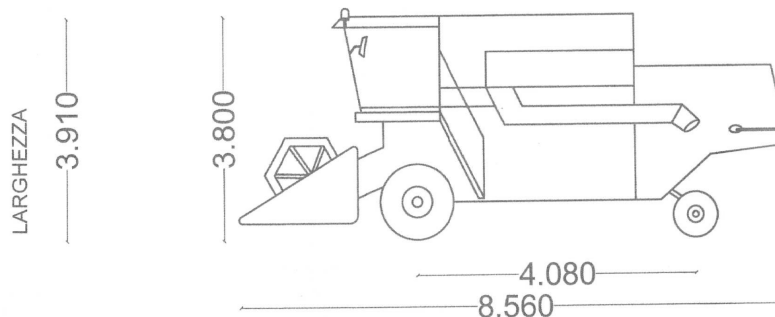
Schema grafico longitudinale della macchina agricola MIETITREBBIA CLAAS S.E. 081 DOMINATOR 198 H, TARGATA AL851V
